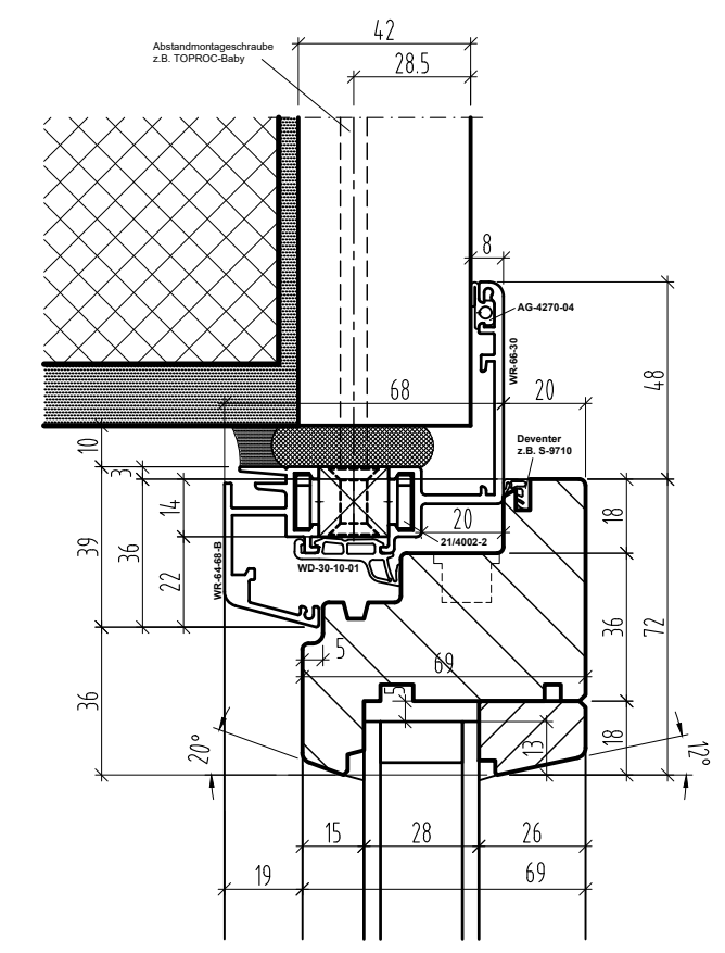
Sirius WR Flügel Sirius H WR-2990-0 Massstab 1:1 1.03.2005 B.W./P.H. 14.03.2005 B.W./P.H. Technische Zeichnung / Technical Drawing
